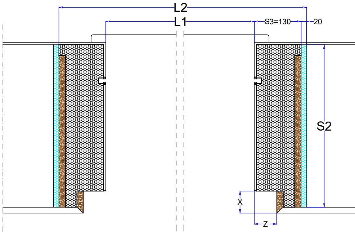
Sezione Orizzontale
