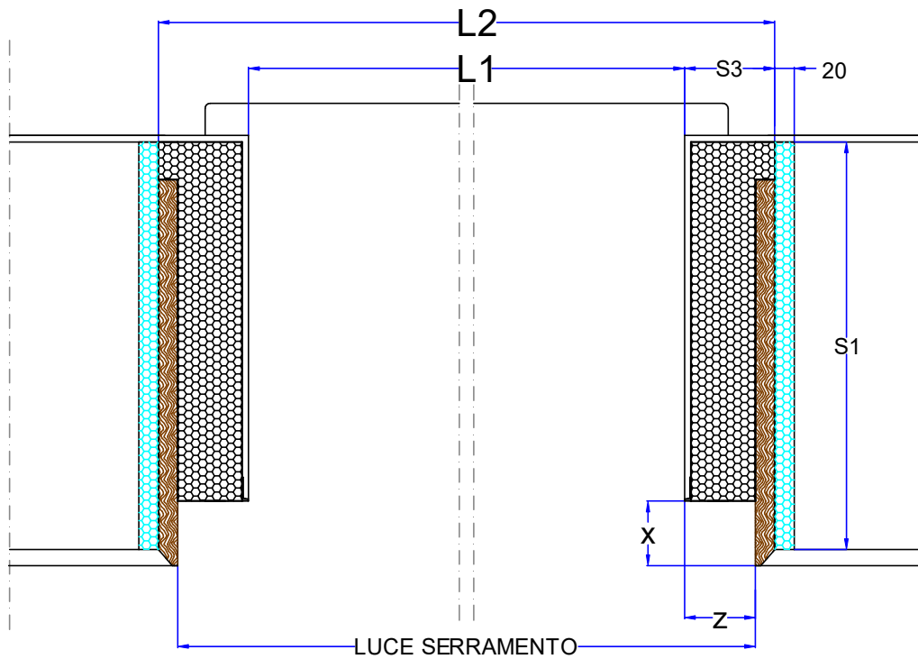
Sezione Orizzontale
