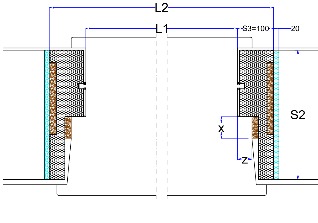
Sezione Orizzontale
