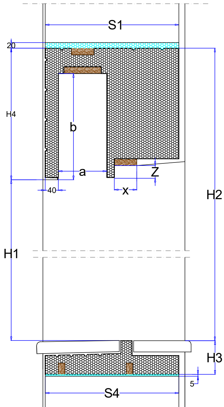
Sezione Verticale
