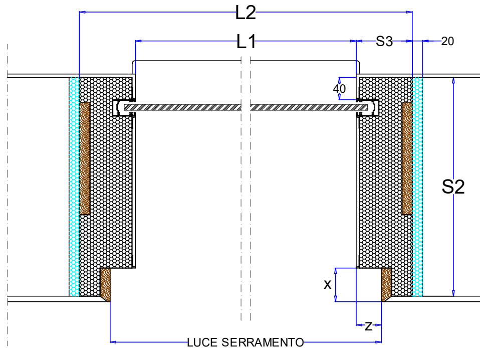
Sezione Orizzontale
