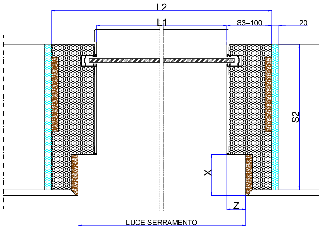
Sezione Orizzontale
