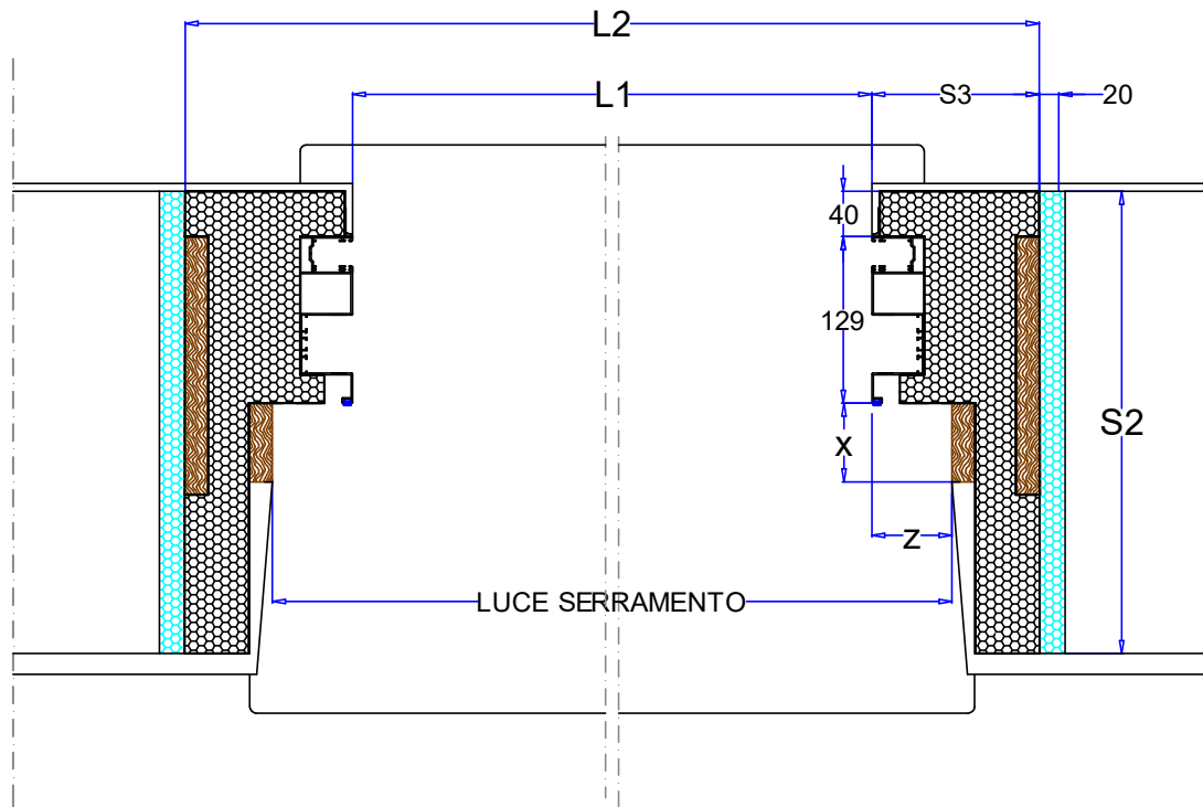
Sezione Orizzontale
