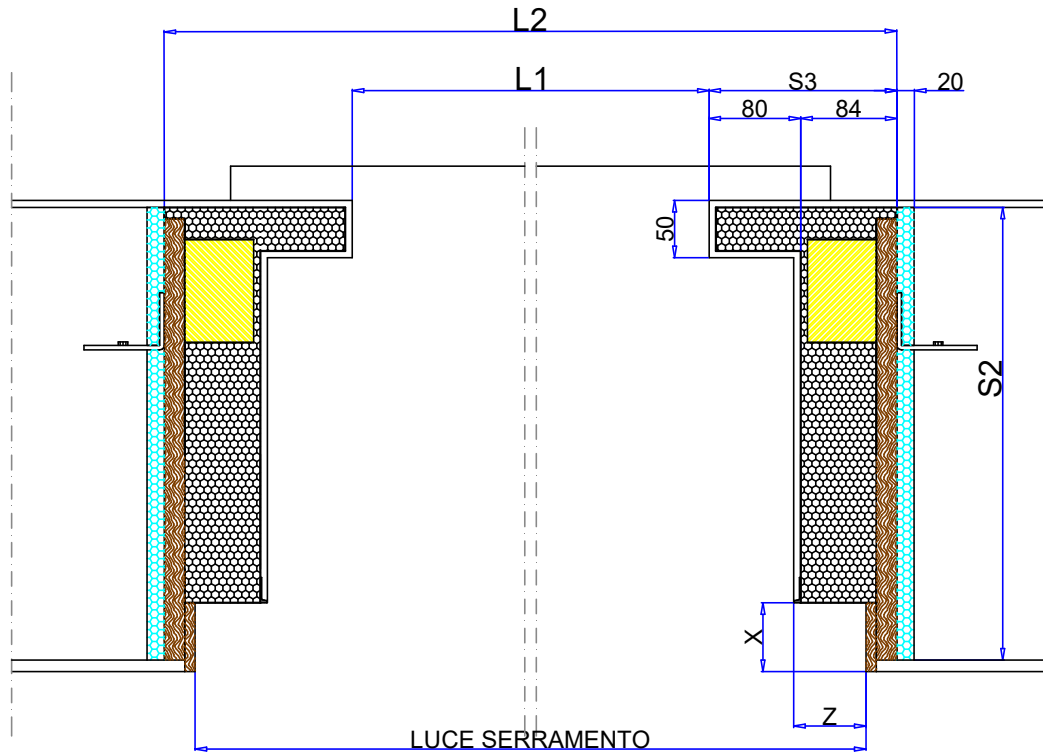
Sezione Orizzontale
