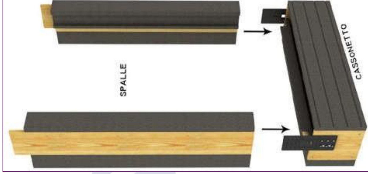
3. ASSEMBLAGGIO DELLE SPALLE CON IL CASSONETTO, AVENDO CURA DI ALLINEARLE AI MARGINI
